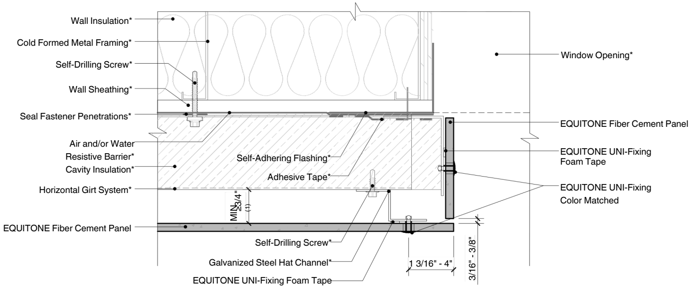
Jamb Detail - Option 1
