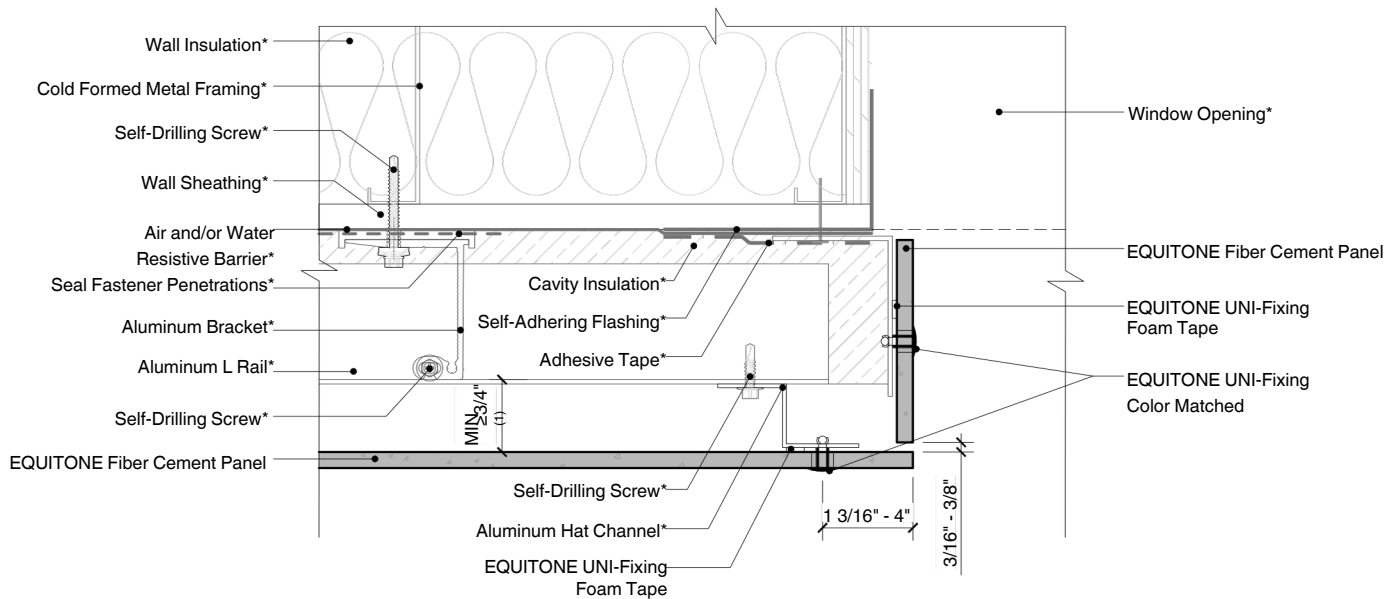
Jamb Detail - Option 1
